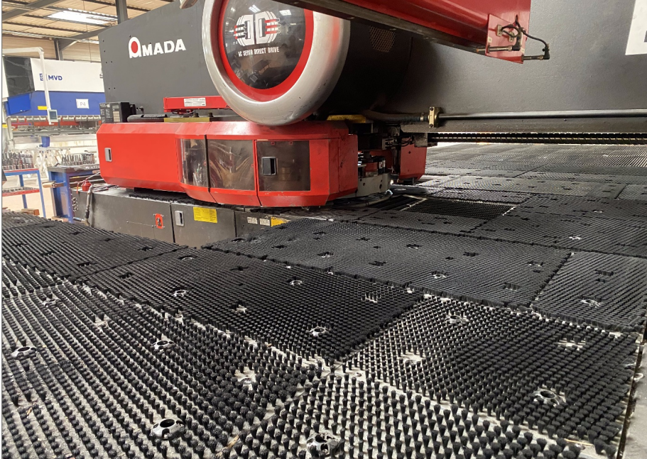
POINCONNEUSE A COMMANDE NUMERIQUE (copie)
