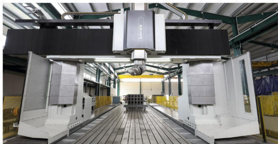
Centre d'usinage gantry - Thera - Zayer (3).webp
