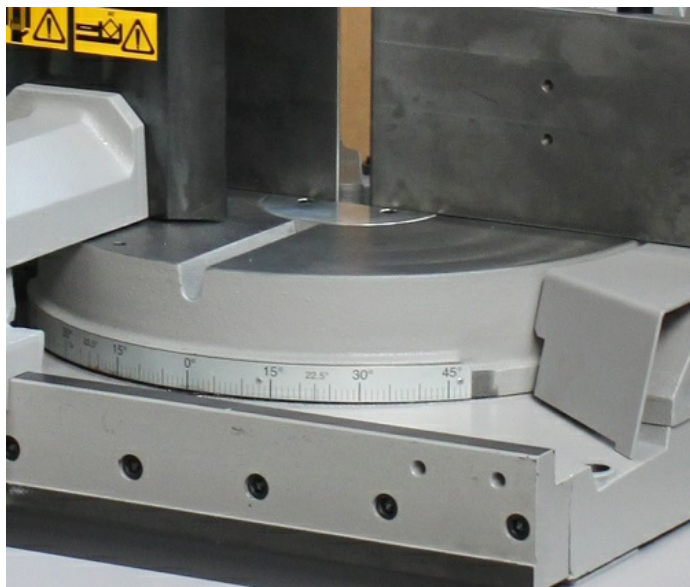
Coupe biseau par base tournante +45°/-60°
