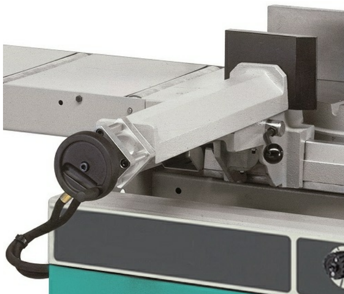
Serrage hydraulique de l'étau
