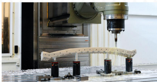
Centre d'usinage - XIOS G XIOS G-MT (7).webp
