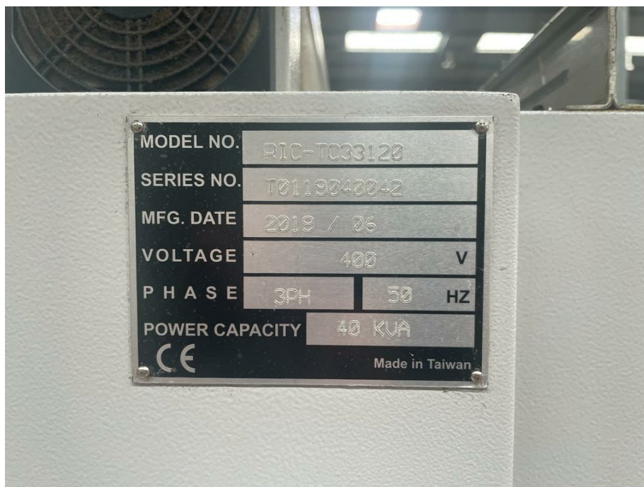
PLAQUE CONSTRUCTEUR
